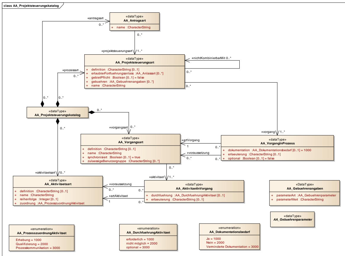
Figure 33: "AA_Projectcontrolcatalogue" (AA_Projektsteuerungskatalog) class diagram
