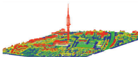
Abb. 18: Telemax Hannover: DOM und ALS-Daten nach Höhen eingefärbt.
