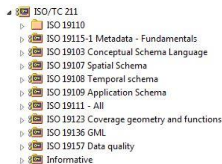
Abbildung 4: Verwendete Teile aus der Normfamilie ISO 19100 (Auszug aus dem UML-Datenmodell)
