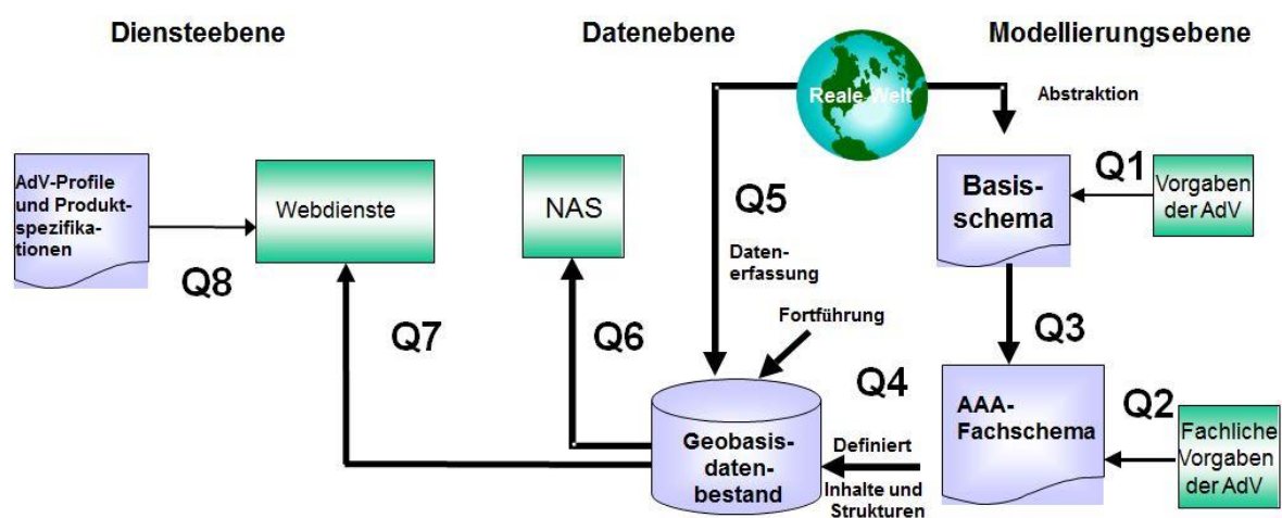
Abbildung 45: Das AdV-Qualitätssicherungsmodell für AAA und Dienste
