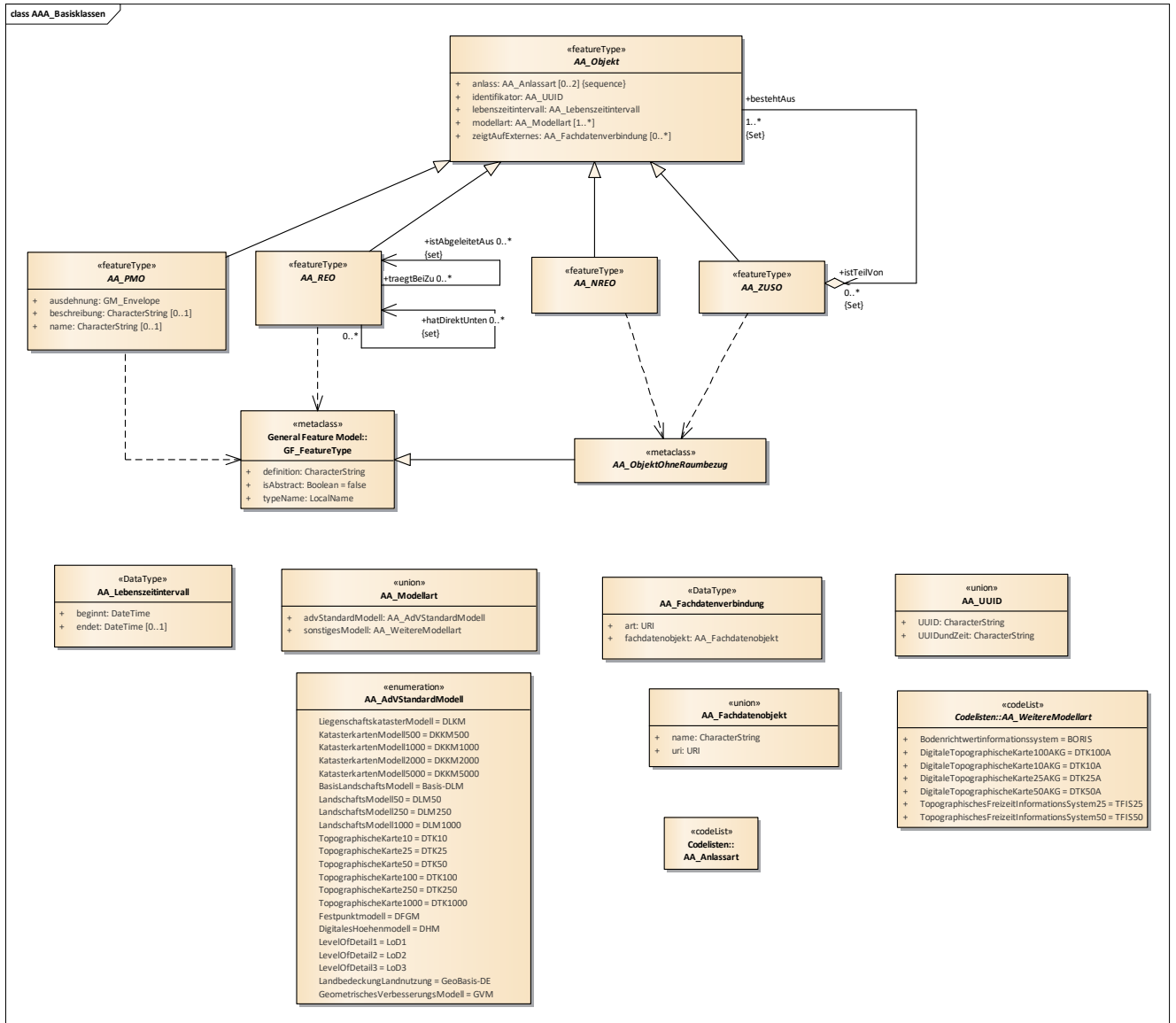
Abbildung 8: Modellierung der AAA-Basisklassen
