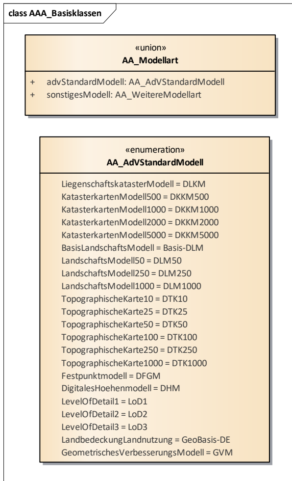
Abbildung 23: Modellarten im Basisschema
