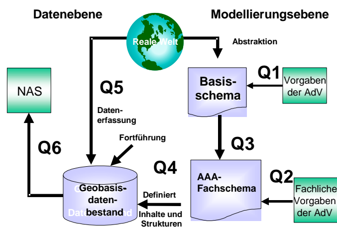
Abbildung 46: Das Qualitätssicherungsmodell des AFIS-ALKIS-ATKIS-Projektes
