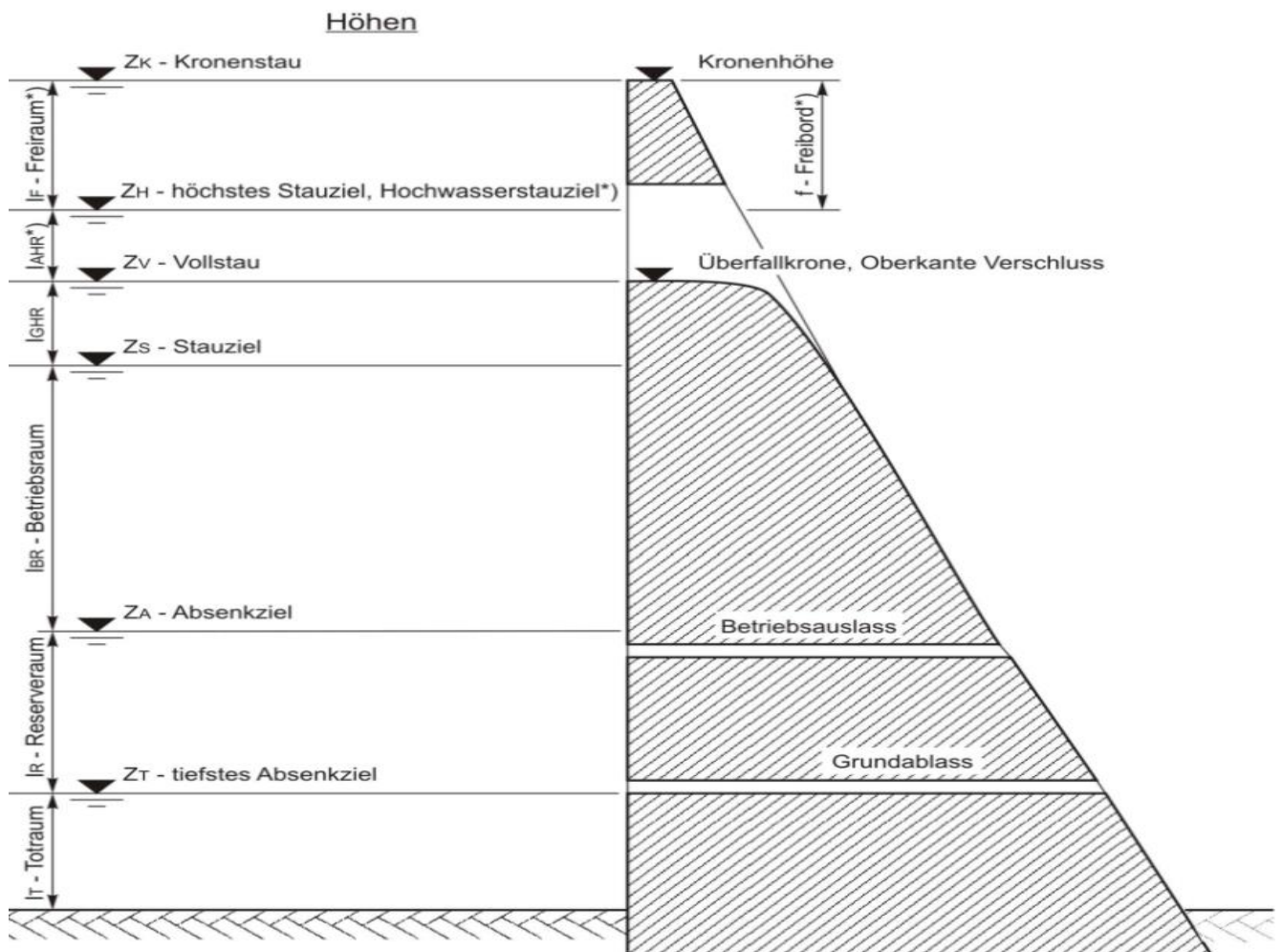
Abbildung 49: Schematische Darstellung der Stau- und Absenkziele bei einem Stausee
