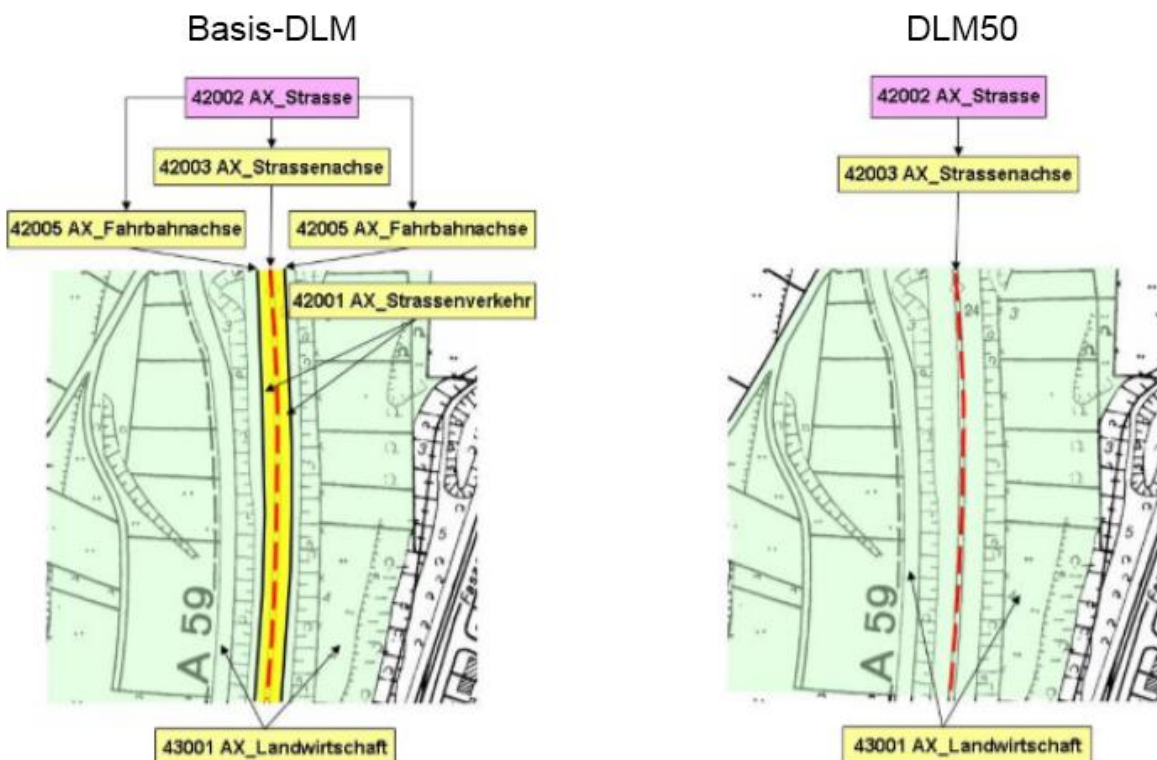
Abbildung 33: Modellierung einer Straße mit physikalisch getrennten Richtungsfahrbahnen im Basis-DLM und DLM50
