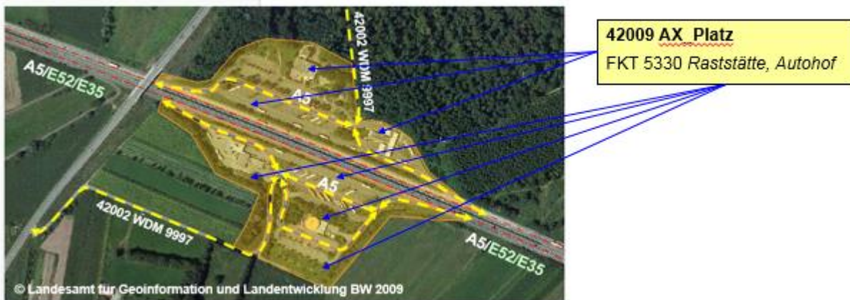
Abbildung 34: Modellierung einer Raststätte
