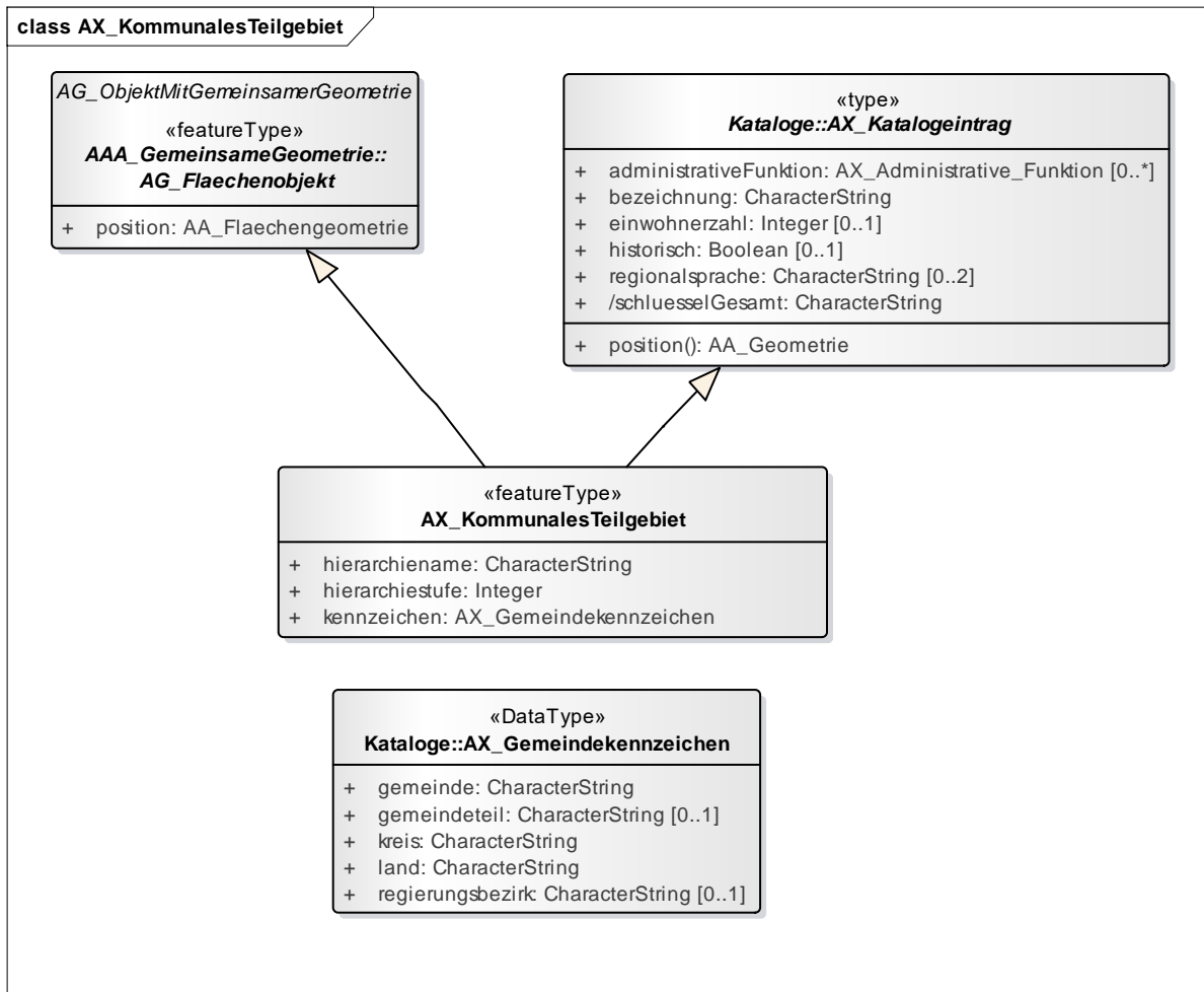
Abbildung 64: Klassendiagramm AX_KommunalesTeilgebiet
