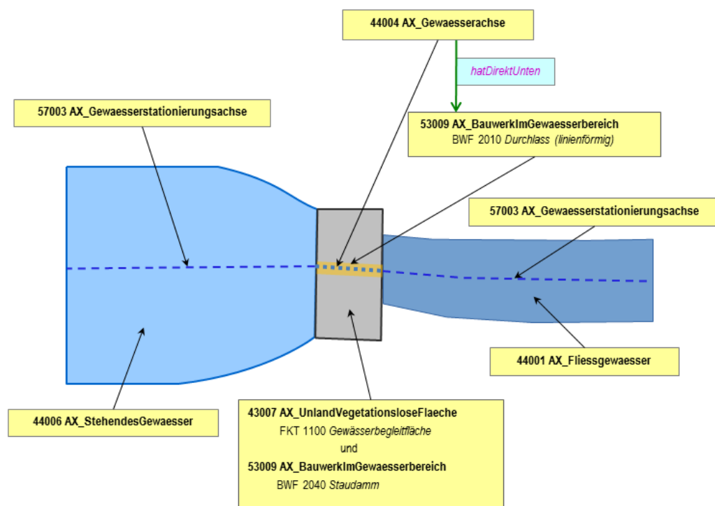
Abbildung 53: Modellierung von Wasserlauf unter Staudamm in linienförmigem Durchlass
