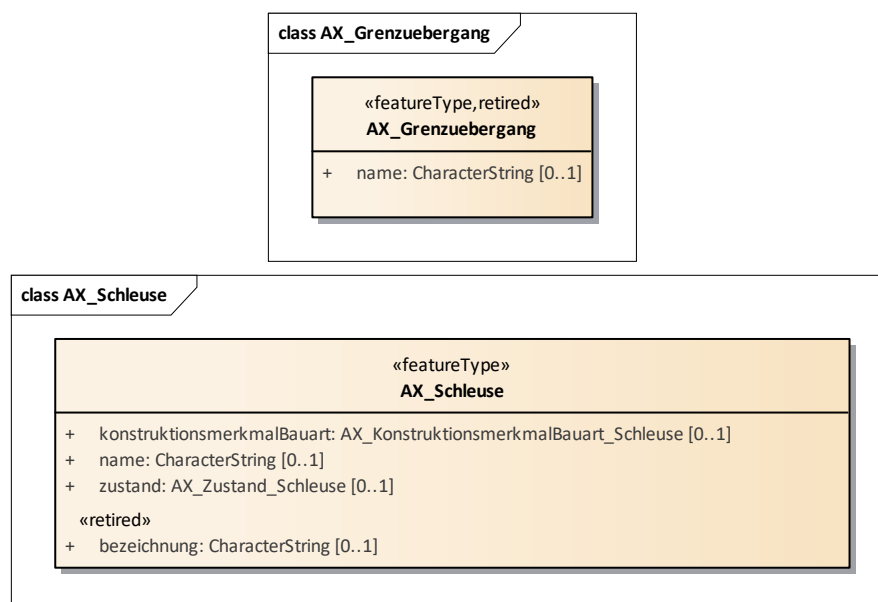
Abbildung 30: Beispiel für eine zurückgezogene Objektart (AX_Grenzebergang) und eine zurückgezogene Attributart (,bezeichnung‘ in AX_Schleuse)
