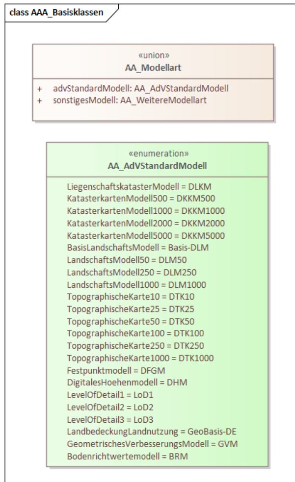
Abbildung 22: Modellarten im Basisschema
