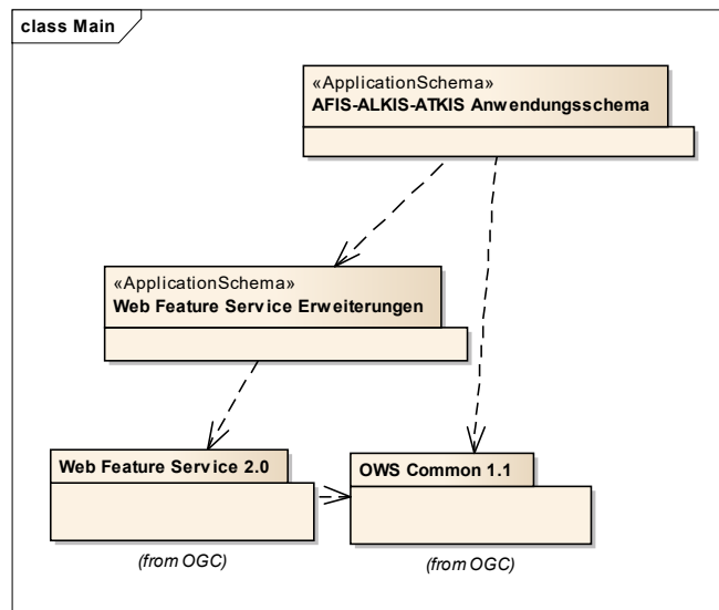
Abbildung 3: Abhängigkeit des AFIS-ALKIS-ATKIS-Anwendungsschemas von den genannten Strukturen aus OGC
