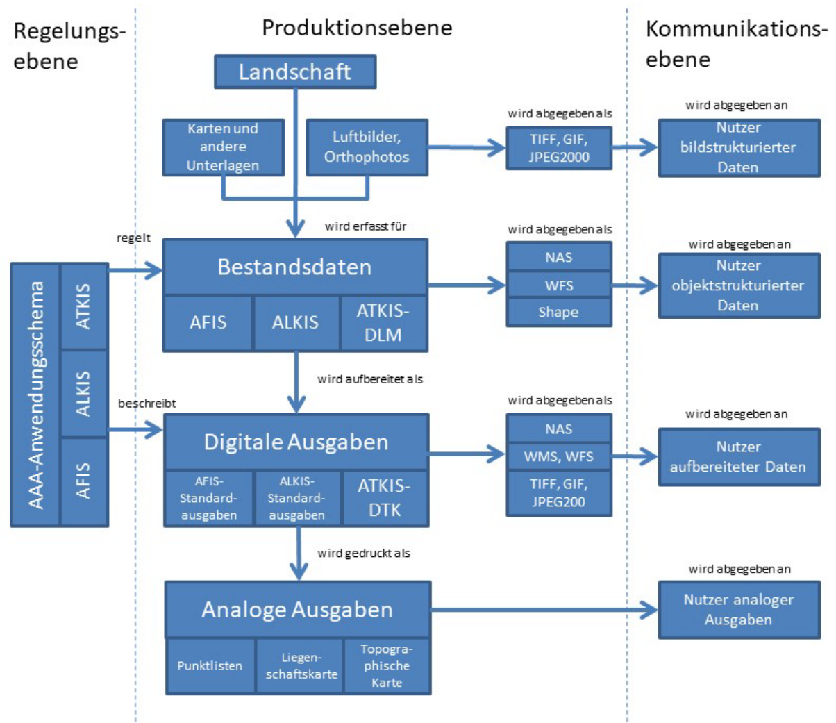
Abbildung 1: Gemeinsames AFIS-ALKIS-ATKIS-Referenzmodell
