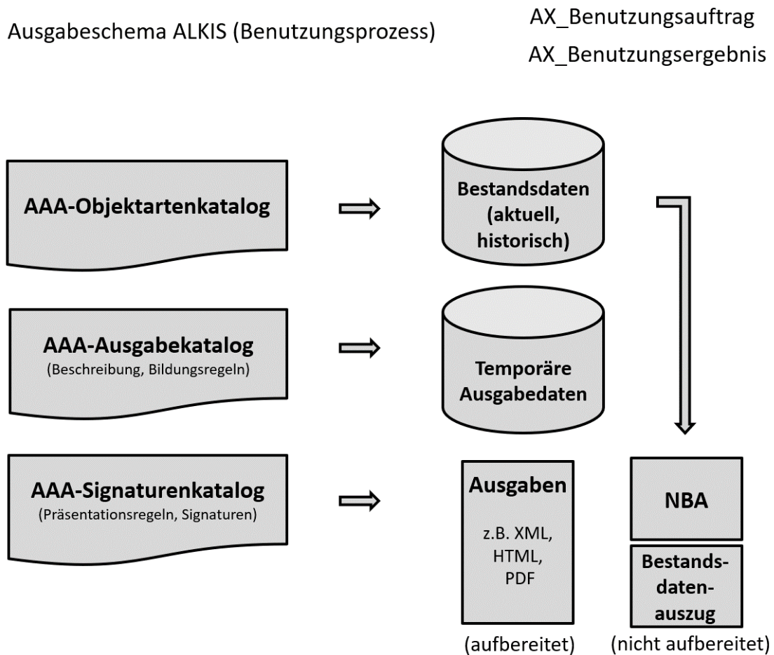
Abbildung 36: Ausgabeschema von ALKIS
