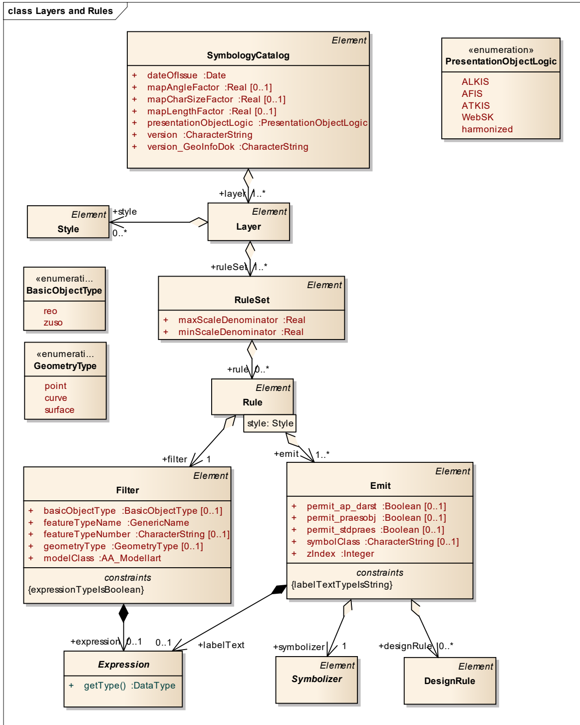
Abbildung 33: Schema SK-Objektmodell
