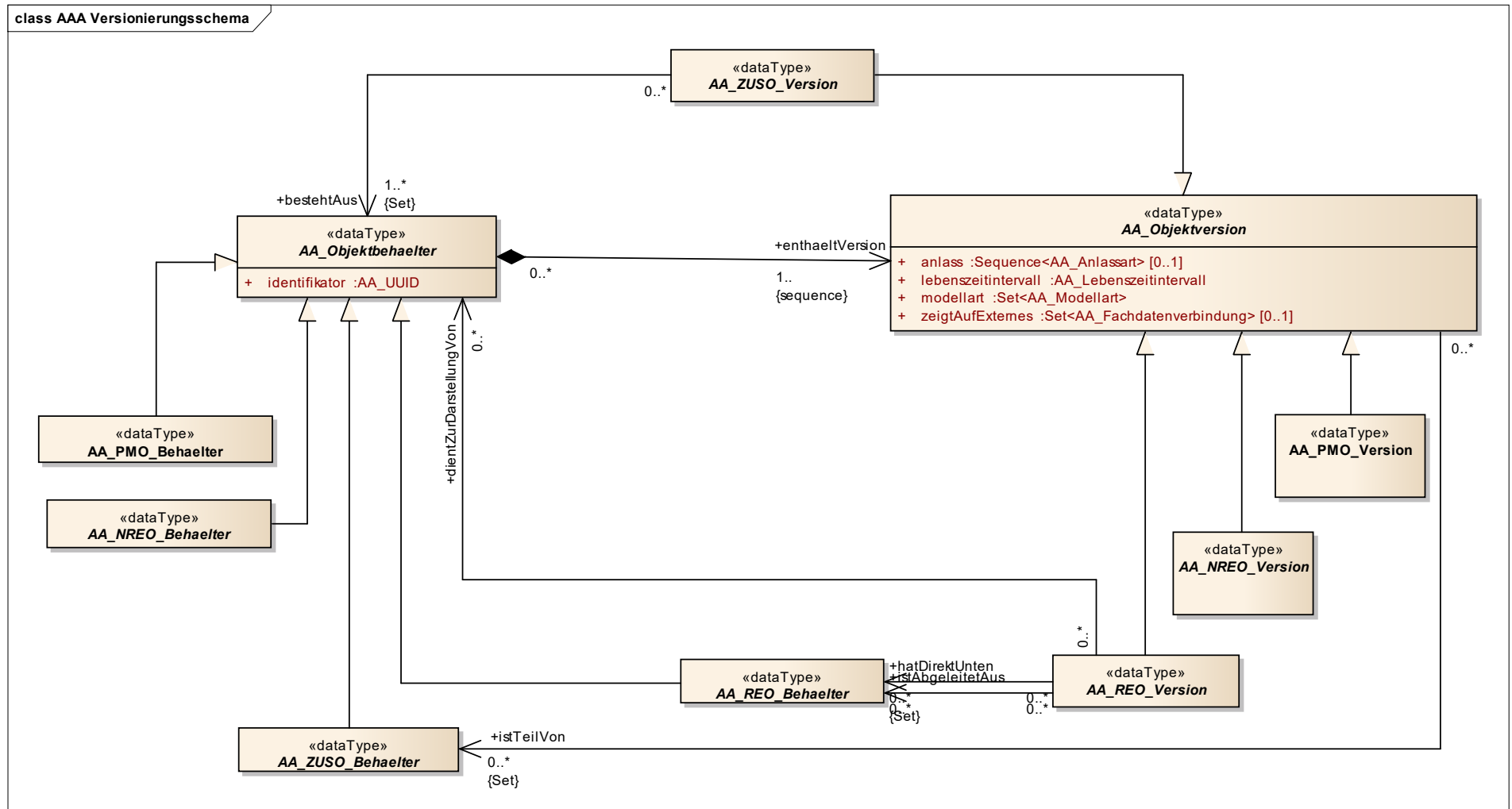
Abbildung 27: Versionierungsschema
