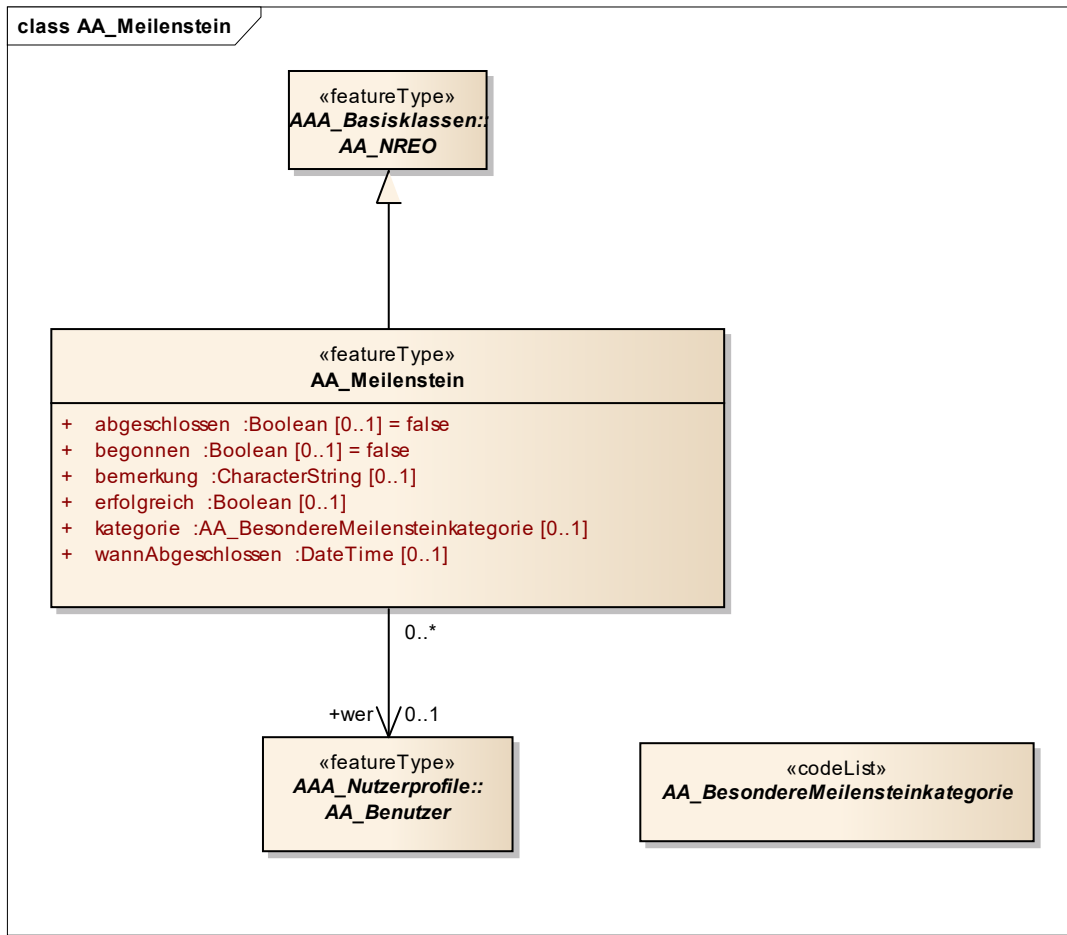
Abbildung 39: Klassendiagramm "AA_Meilenstein"
