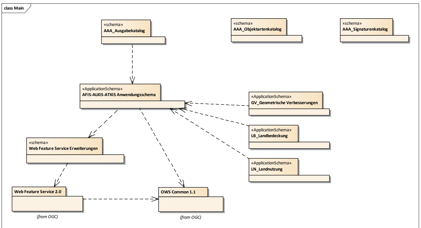
Abbildung 5: Die Bestandteile des AFIS-ALKIS-ATKIS-Anwendungsschemas
