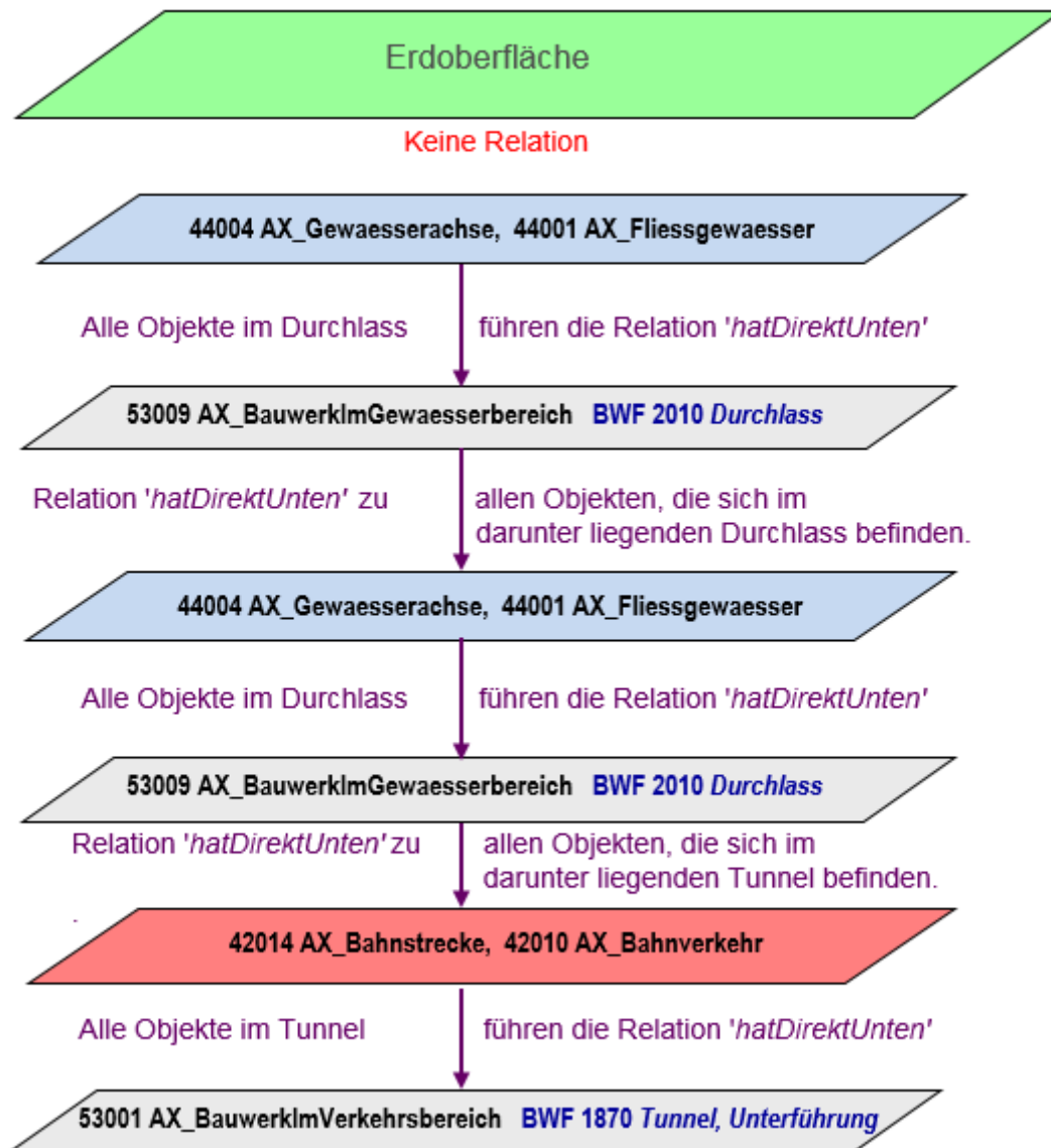
Abbildung 19: Vertikale Abbildung der Landschaft unter der Erdoberfläche
