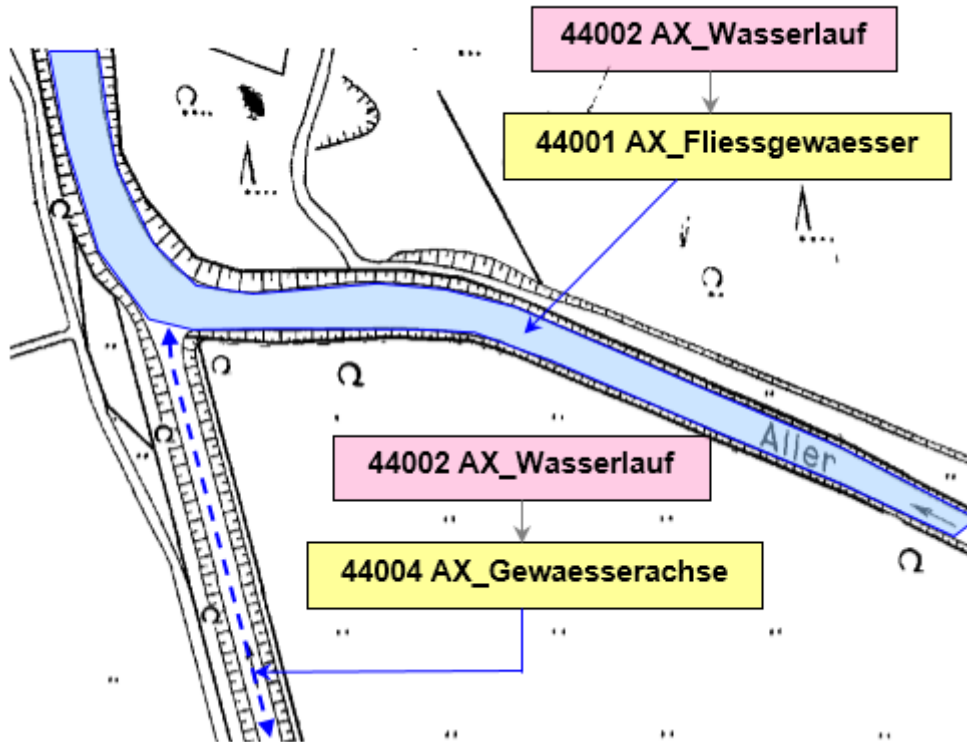
Abbildung 40: Modellierung von Wasserläufen
