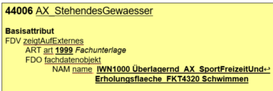
Abbildung 41: Beispiel für die Belegung der weiteren Nutzung „Schwimmen“ im Attribut „zeigtAufExternes“
