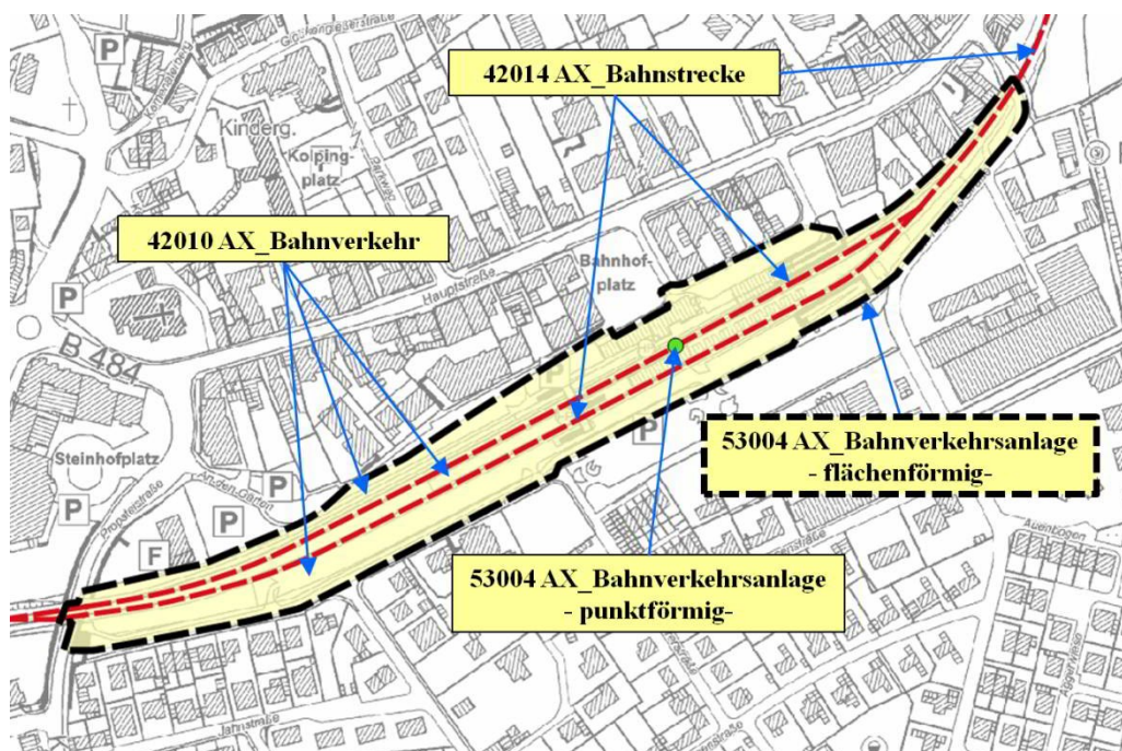
Abbildung 38: Modellierung mehrerer Bahnstrecken
