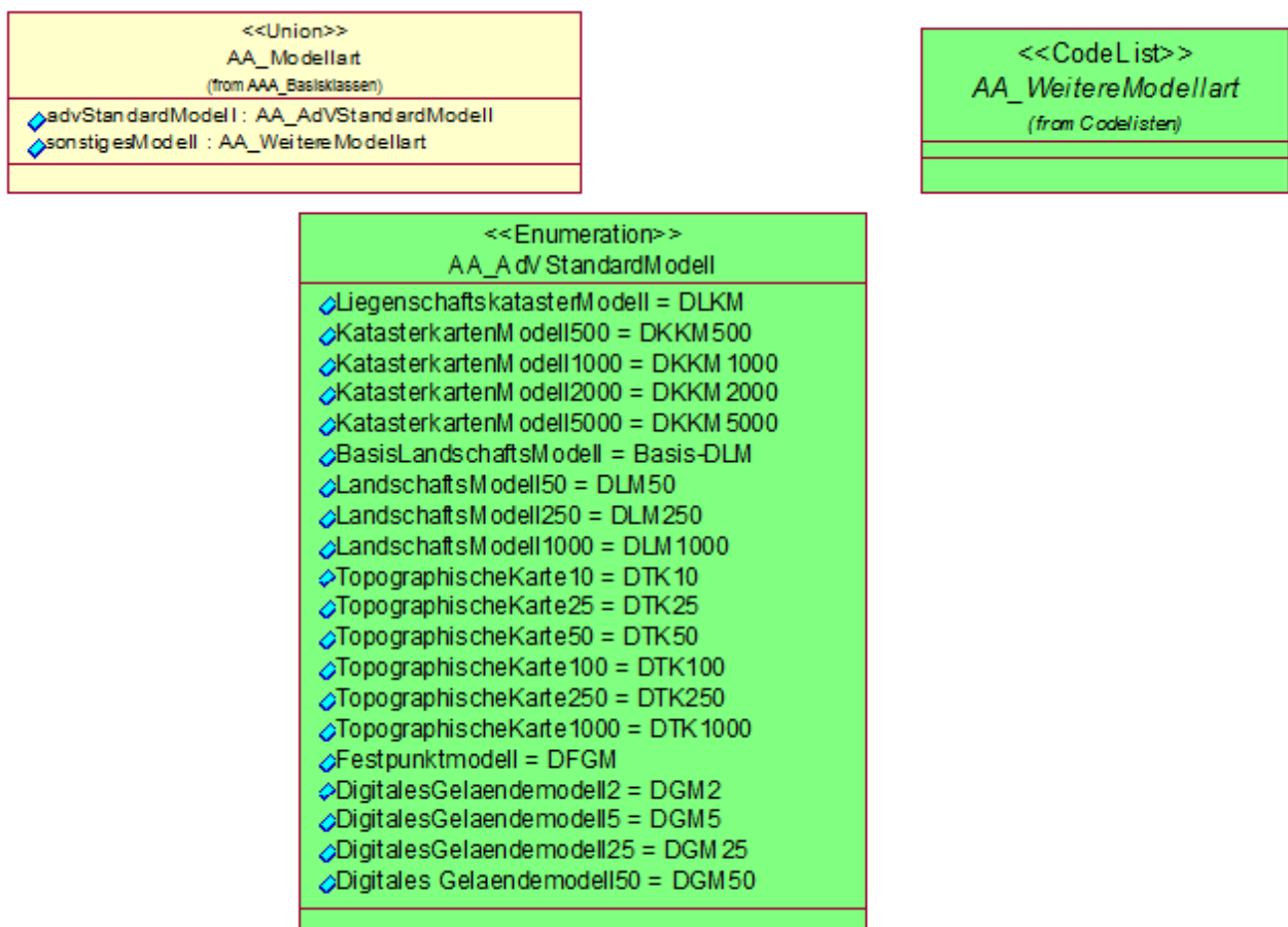
Abbildung 21: Modellarten im Basischema
