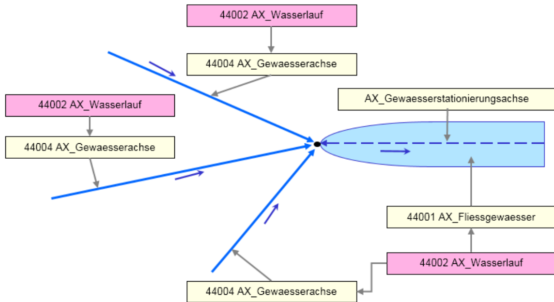
Abbildung 42: Modellierung von Wasserläufen unter Beachtung der Fließrichtung
