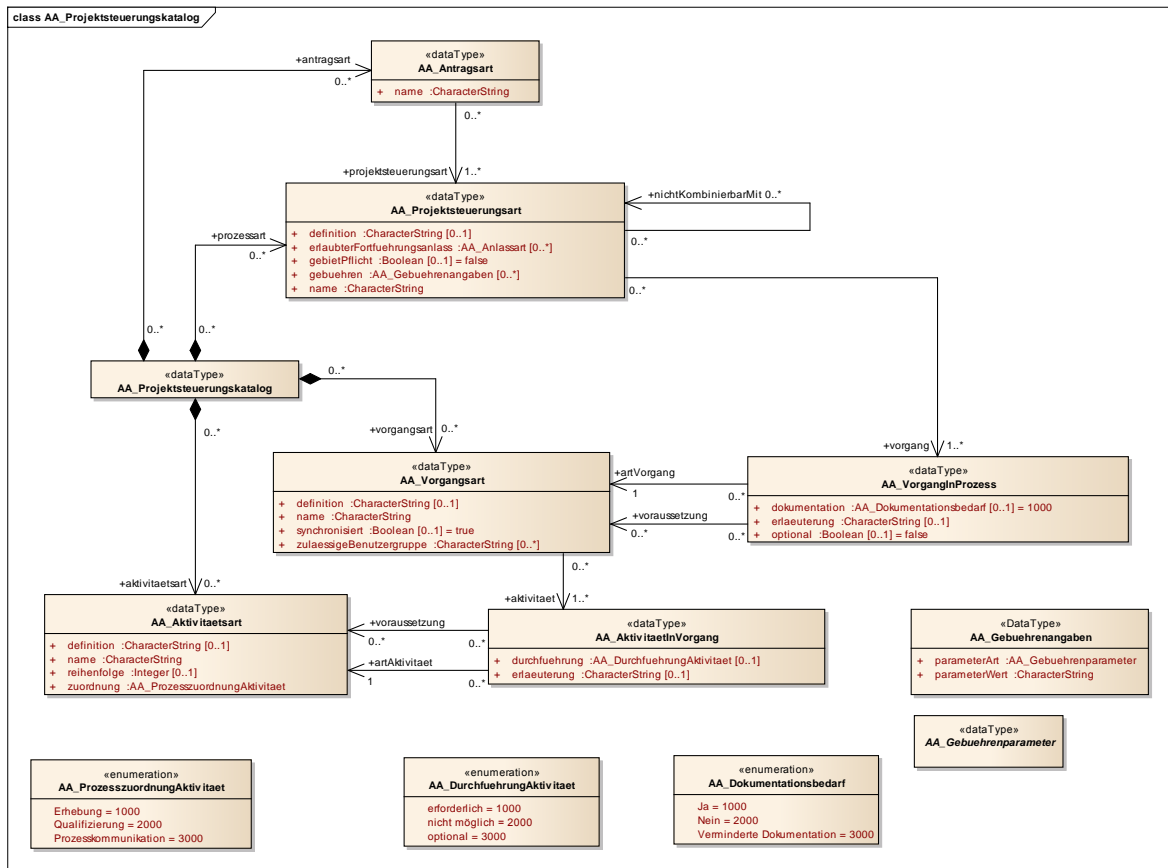
Abbildung 37: Klassendiagramm "AA_Projektsteuerungskatalog"
