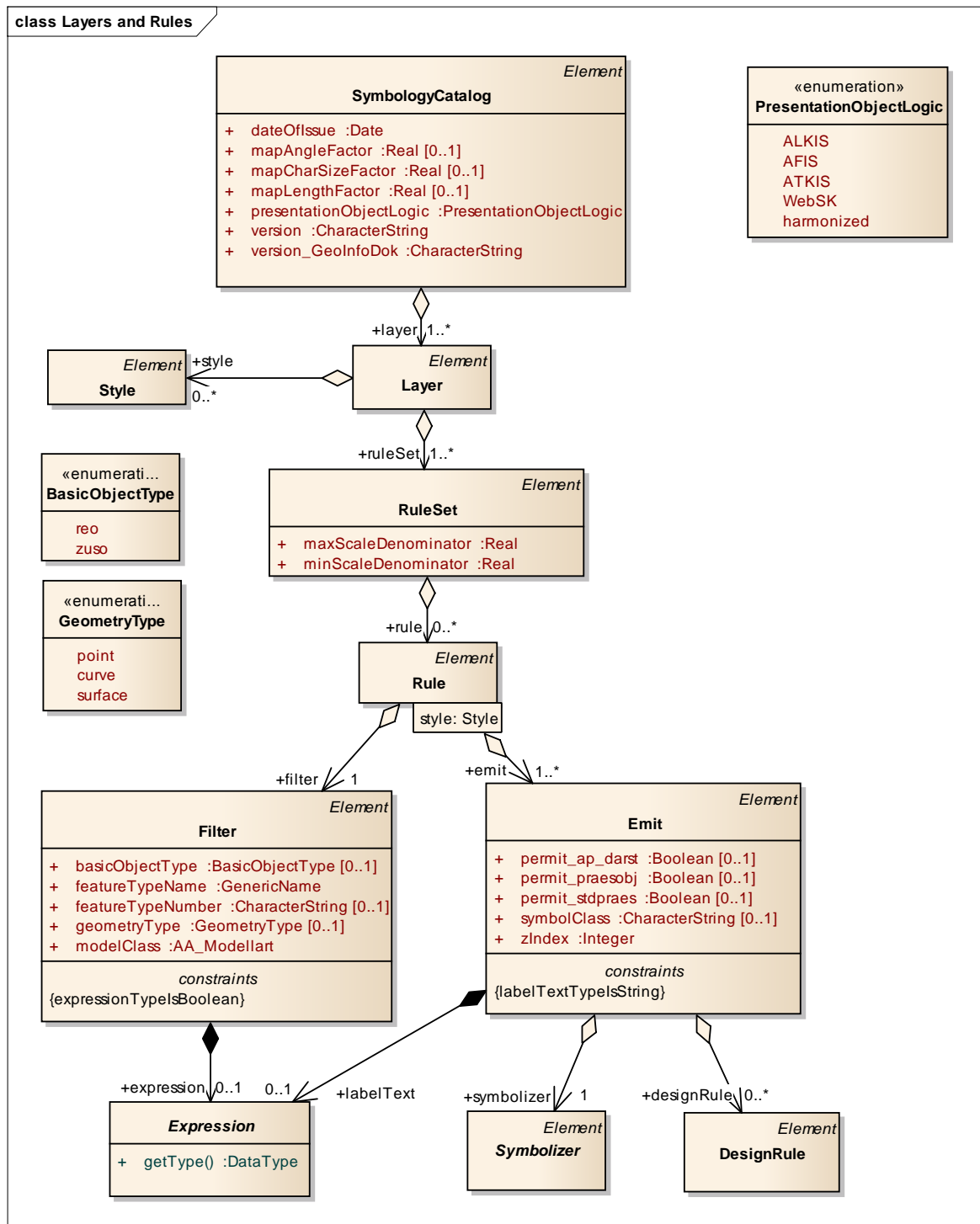
Abbildung 32: Schema SK-Objektmodell
